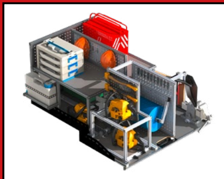
23 Supporto per motosega su Pianale estraibile sinistro/ chainsaw bracket on sliding tray left
